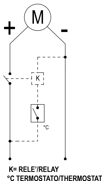
COLLEGAMENTO ELETTRICO 12-24V DC 12-24V DC ELECTRIC WIRING
