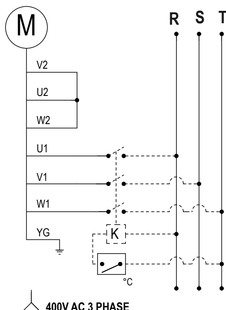
COLLEGAMENTO ELETTRICO 400V AC TRIF. 400V AC THREEPHASE ELECTRIC WIRING
